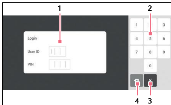
Fig. 8-9: L'écran Login
