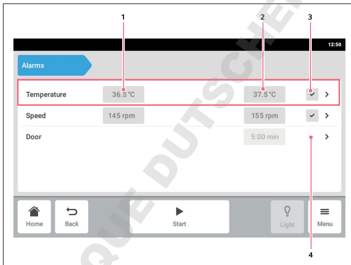
Fig. 8-4: L'écran Alarmes
