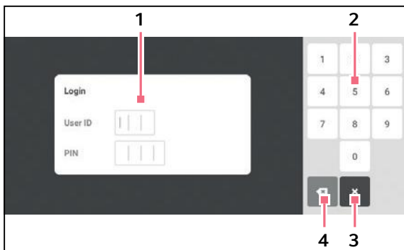
Fig. 8-9: L'écran Login
