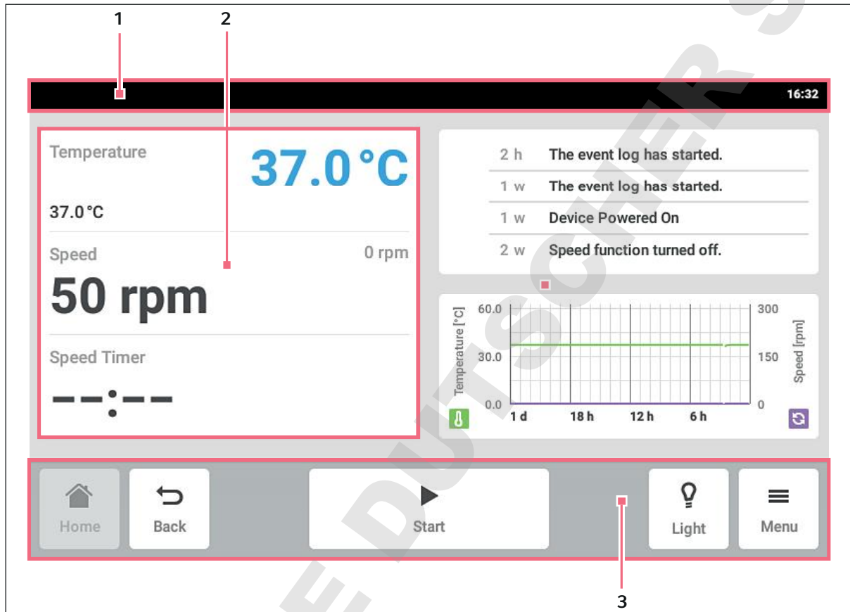
Fig. 6-1: Écran d'accueil
