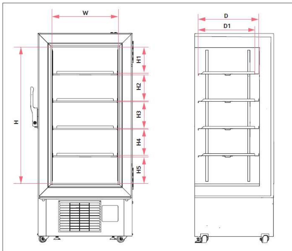
Fig. 10-2: Dimensions internes CryoCube F440n et CryoCube F440h
