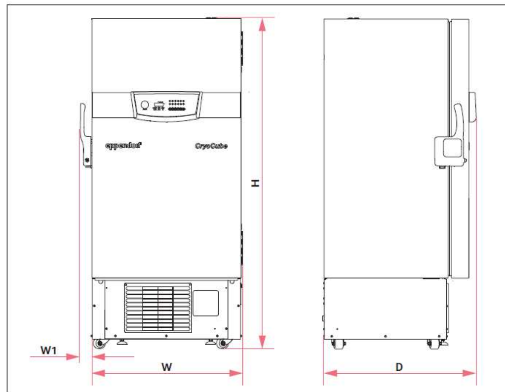
Fig. 10-1: Dimensions externes CryoCube F440n et CryoCube F440h
