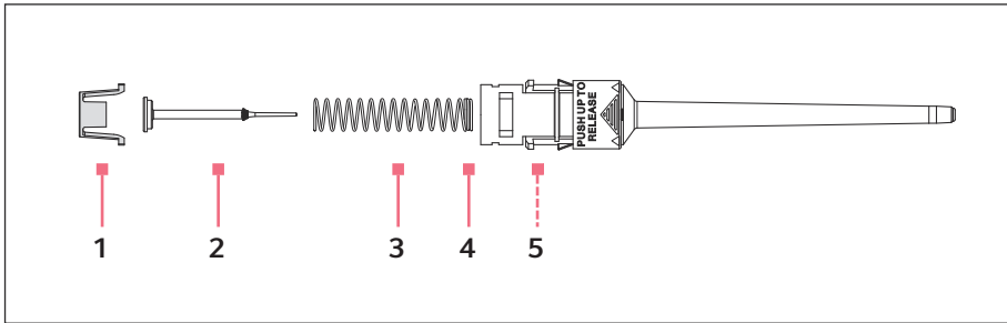
Fig. 7-1 : Partie basse de la pipette monocal ≤ 1000 µL
