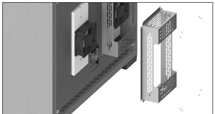
III. 31 Capot du module de refroidissement Peltier à l'arrière de l'appareil
