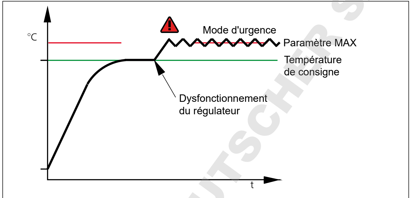
III. 20 Schéma du fonctionnement du dispositif de sécurité TWW
