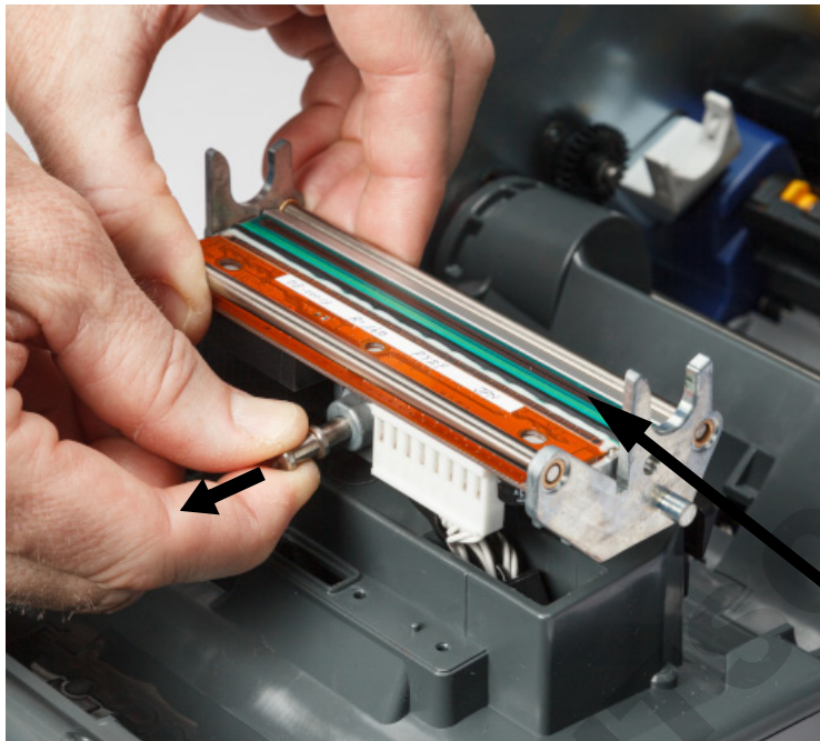
Élément chauffant
