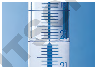
Indication du ménisque par la bande photophore d'une burette.
