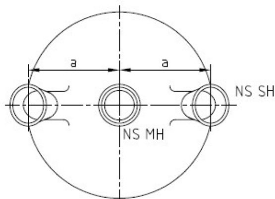
Draufsicht Dreihals-Rundkolben
