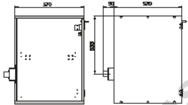
Vue latérale
