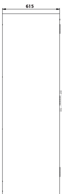
Vue latérale
