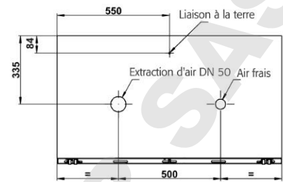
Vue arrière UB90.060.110.050.2T
