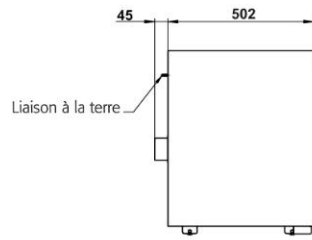
Vue de côté UB90.060.110.050.2T
