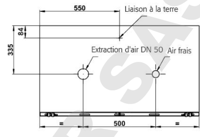
Vue arrière UB90.060.110(.050).2S
