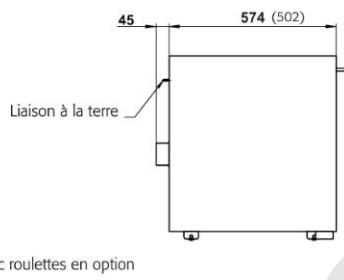
Vue de côté UB90.060.110(.050).2S
