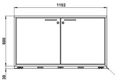
Vue de face UB90.060.110(.050).2S
