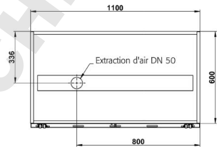
Vue de dessus SL.060.110.UB.2T
