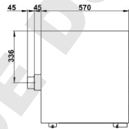
Vue de côté SL.060.140.UB.3T
