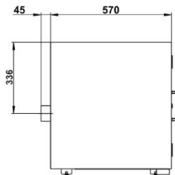
Vue de côté SL.060.059.UB.T(R)
