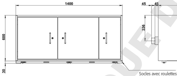
Vue de face SL.060.140.UB.3T
