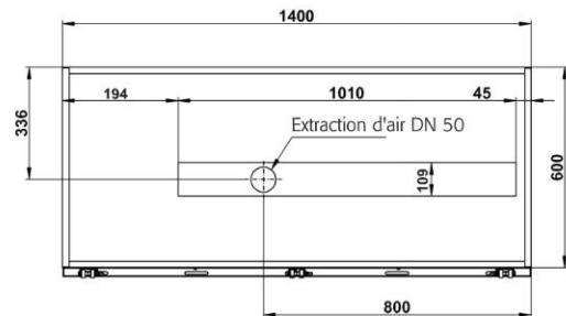
Vue de dessus SL.060.140.UB.3T
