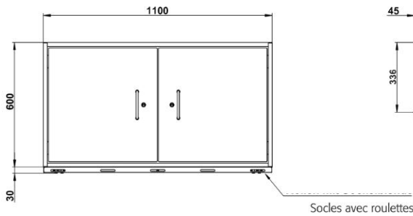
Vue de face SL.060.110.UB.2T
