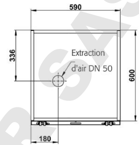
Vue de dessus SL.060.059.UB.T(R)
