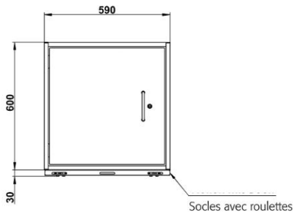
Vue de face SL.060.110.UB.2T
