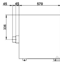
Vue de côté SL.060.110.UB.2T
