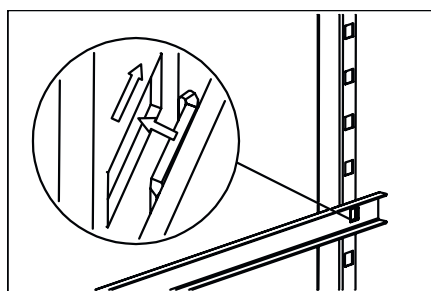
Fig. 39 : Emboîter le rail d'appui à l'arrière
