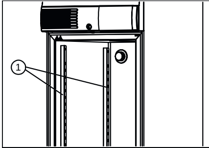
Fig. 211 : Rails d'arrêt
