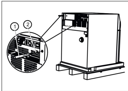
Fig. 21 : Monter la barre métallique
