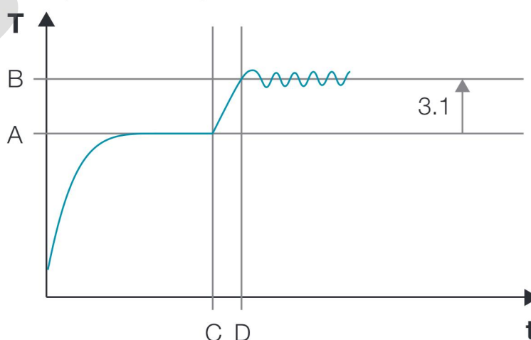
Fig. 153 : Diagramme « Contrôle de température » classe 3.1
