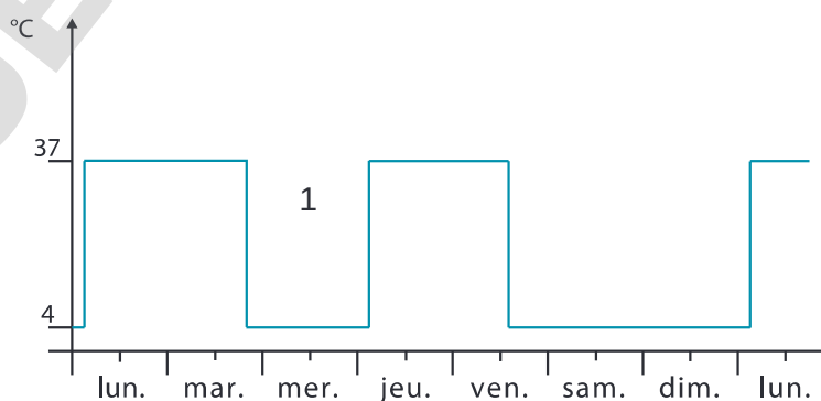
Fig. 221 : Diagramme « Baisse de température avec fonction jours fériés (sur l'exemple de mercredi) »
