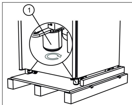
Fig. 18 : Visser les éléments de mise à niveau
