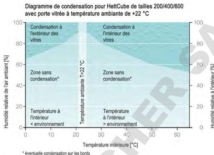
Fig. 9 : Diagramme de condensation
