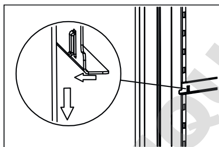
Fig. 40 : Accrocher la partie avant
