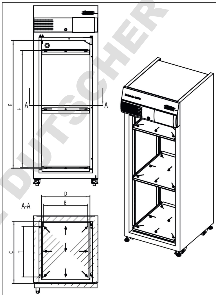
Fig. 215 : Volume utile
