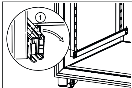
Fig. 45 : Tourner l'avant du rail télescopique
