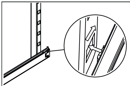
Fig. 42 : Emboîter le rail télescopique à l'arrière
