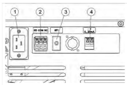
Fig. 26 : Autres branchements
