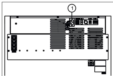
Fig. 25 : Raccord alimentation en courant
