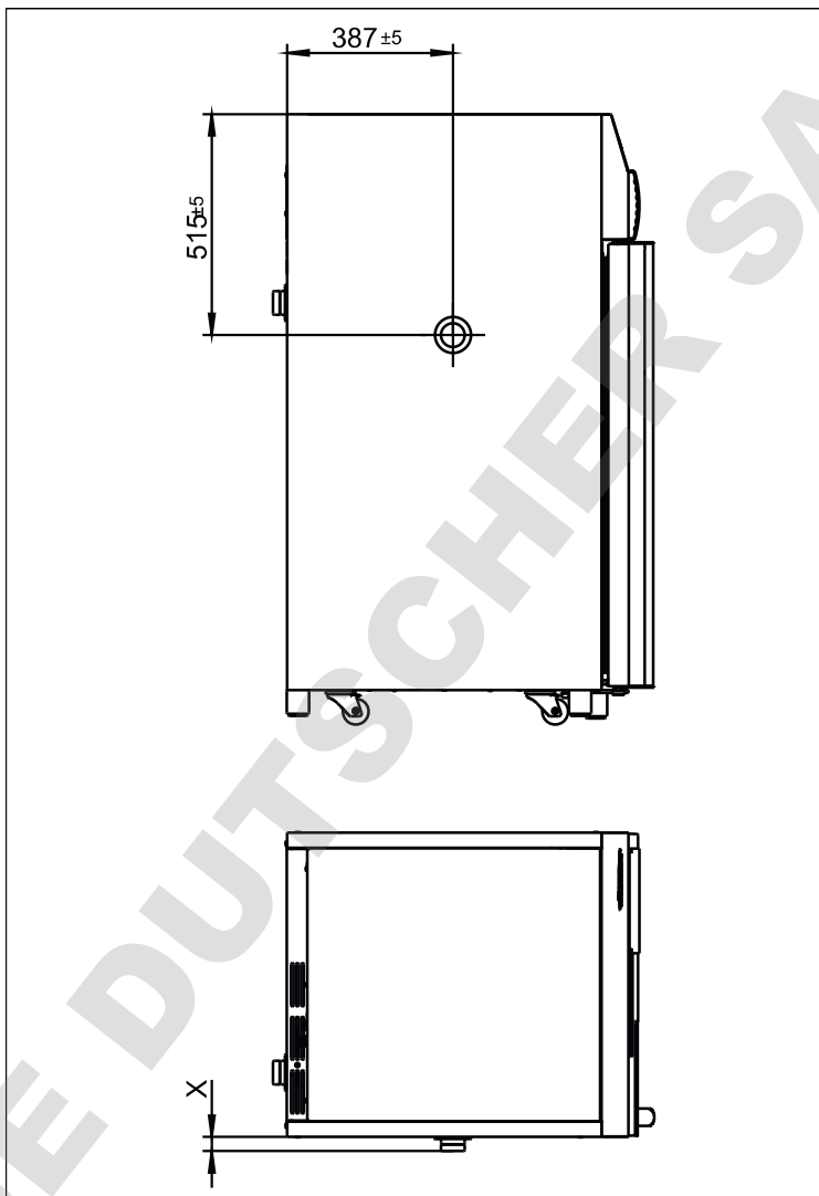
Fig. 218 : Dimensions « Passage de câble sur le côté »
