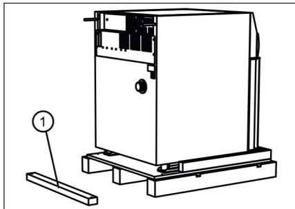
Fig. 22 : Poutre avant sur le sol
