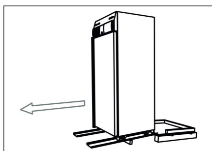
Fig. 19 : Faites rouler l'incubateur sur les rails métalliques pour le descendre
