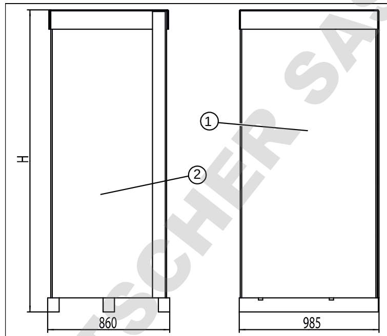
Fig. 14 : Dimensions emballage pour le transport
