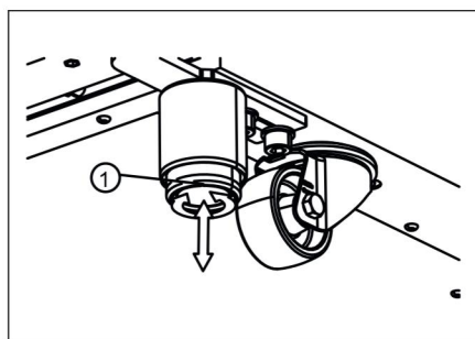
Fig. 24 : Mise à niveau de l'incubateur
