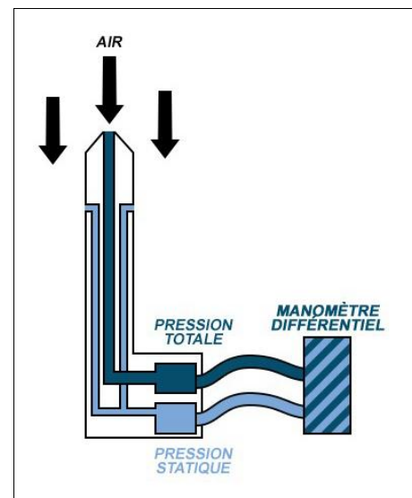
Schéma du tube de Pitot
