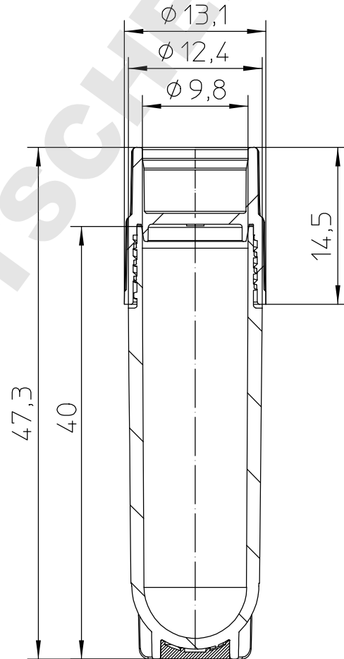
Schnitt A-A
