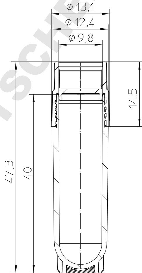
Schnitt A-A
