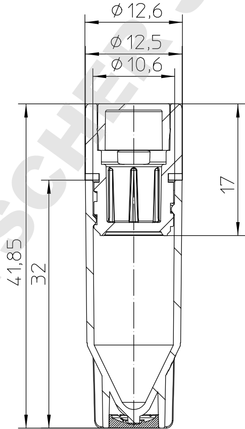
Schnitt A-A
