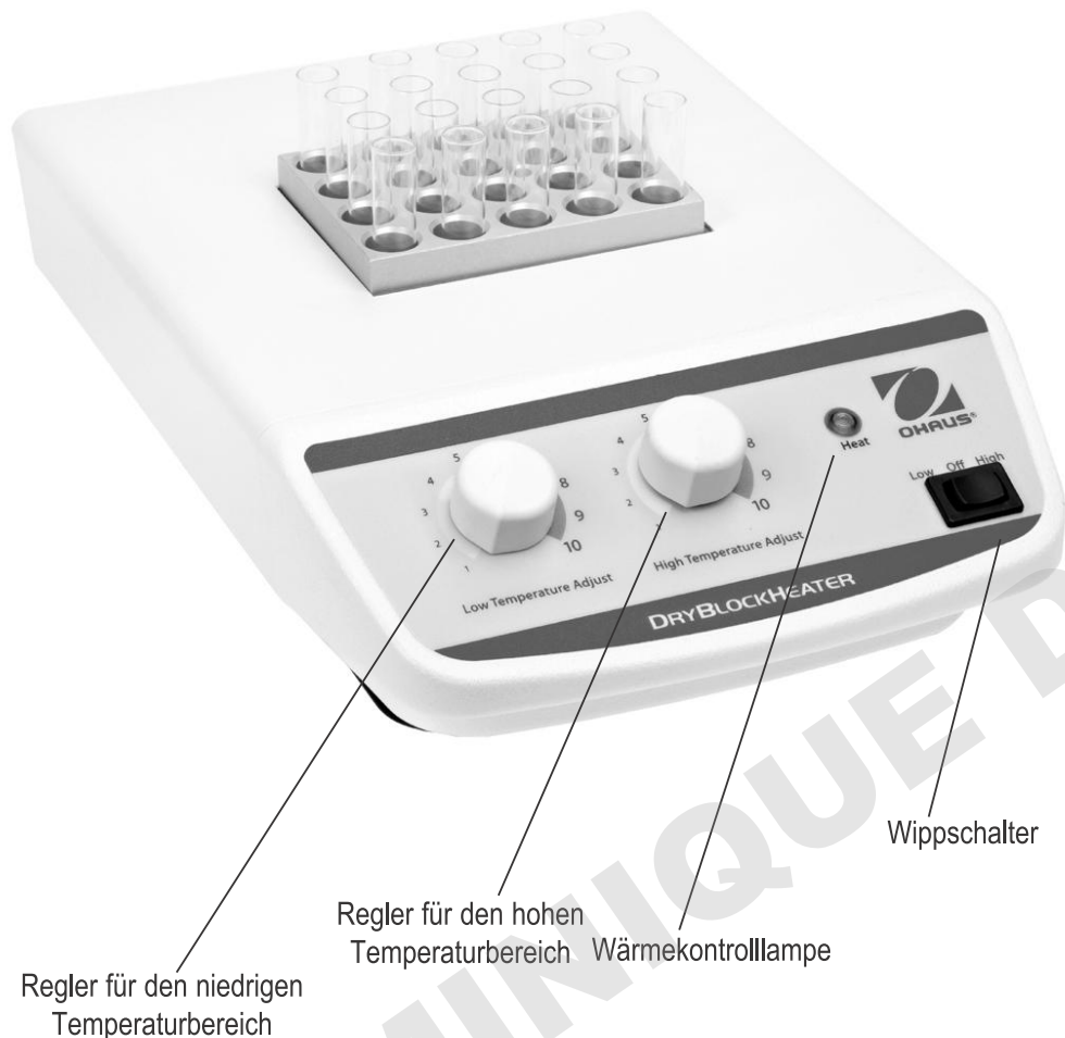
Ohaus 1-Block Heizblockthermostat, analog, mit Modulblöcken und Röhrchen
