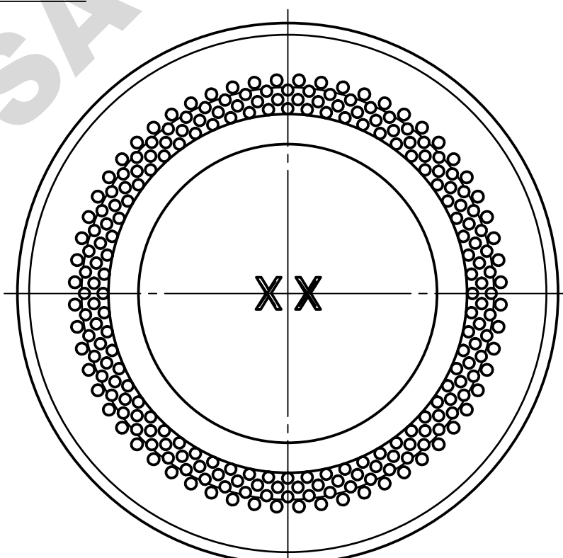
4 Reihen Noppen je Teilkreis 4 rows of knobs per pitch circle
