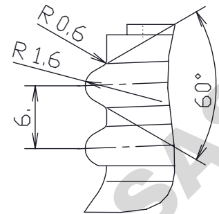
Einzelheit X M 2:1
