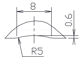
Nahteinzug M 2:1
