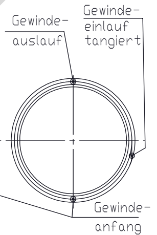
Einzelheit X M 2:1
