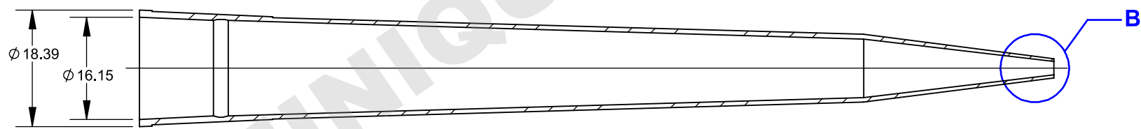
SECTION A-A SCALE: 1.2 : 1
