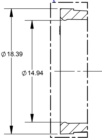
DETAIL A SCALE: 3 : 1
