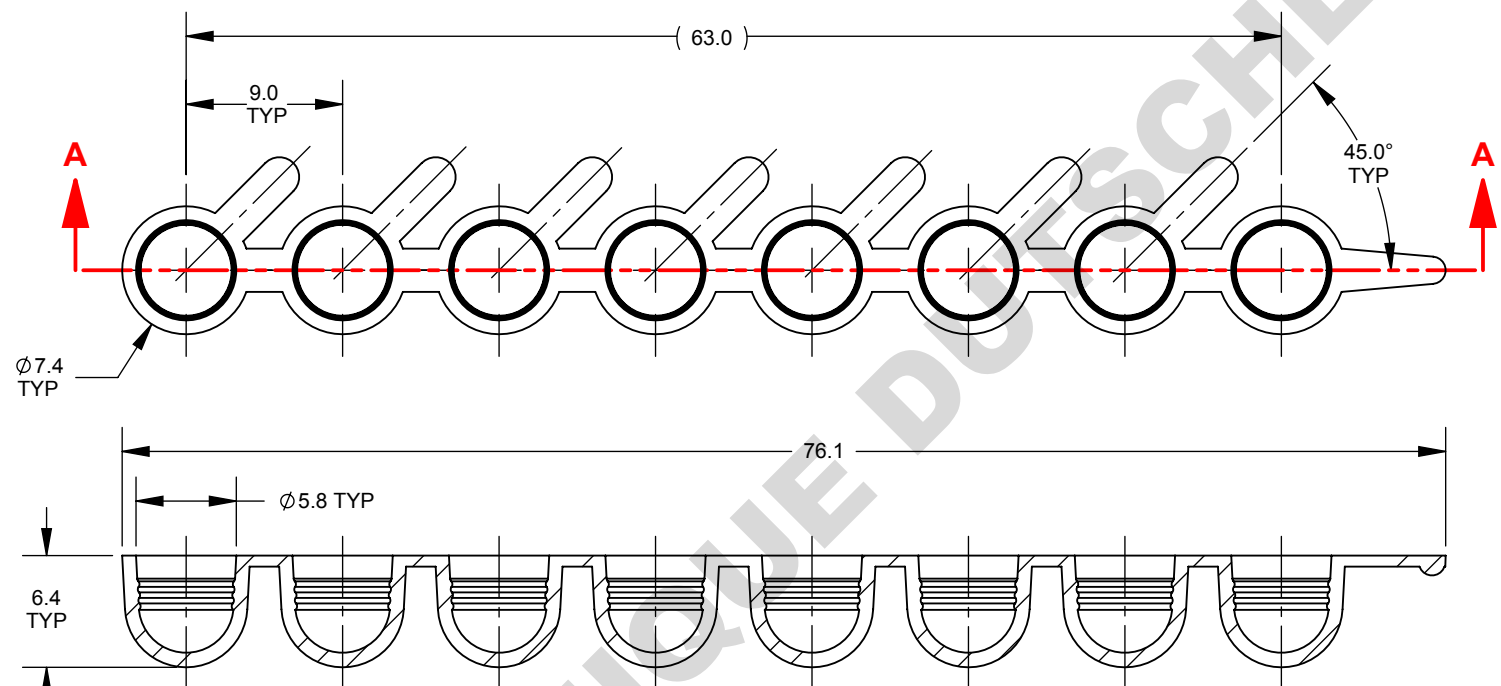
SECTION A-A SCALE: 2.3 : 1
