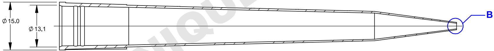
SECTION A-A
