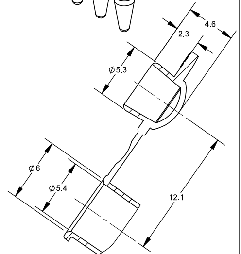
DETAIL B SCALE: 3.8 : 1 TYP
